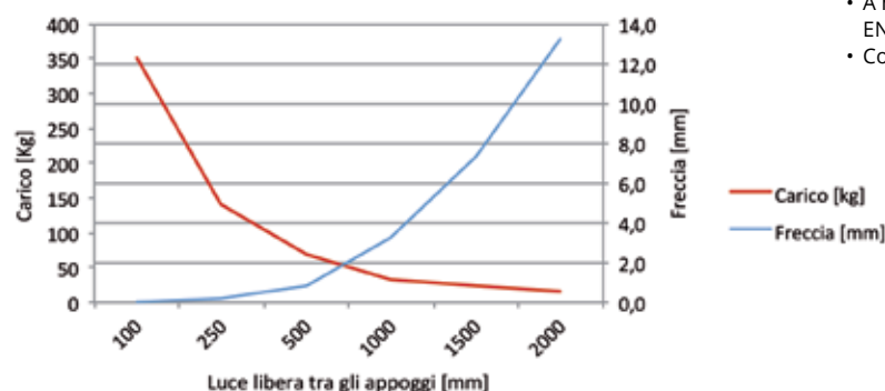
carico max.concentrato in mezzeria
