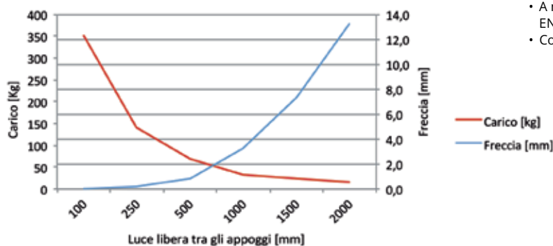
carico max.concentrato in mezzzeria
