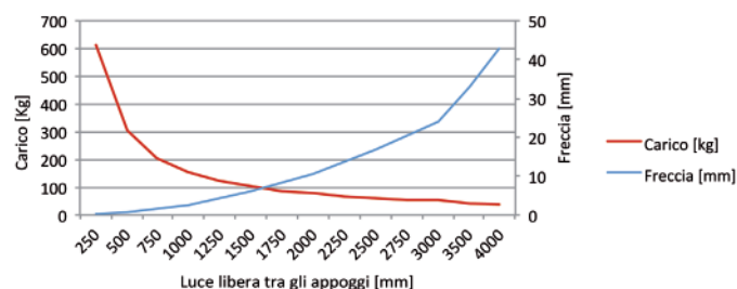
carico max.concentrato in mezzaria
