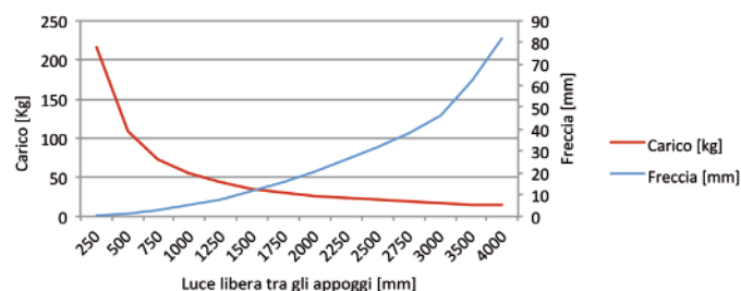
carico max.concentrato in mezzzeria
