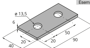
Esempio di montaggio / Assembly example
